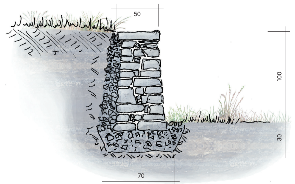
Stützmauer
