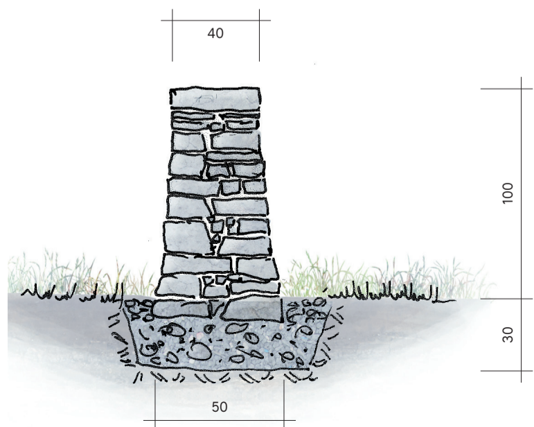
Gartenmauer
